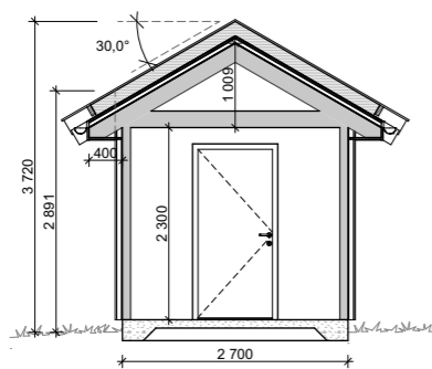
Snitt A
